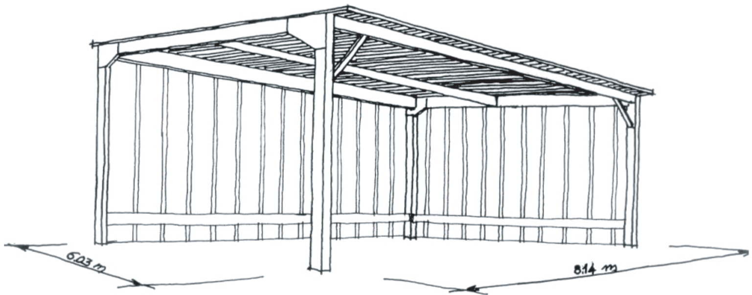
Modèle A86 / 49.08 m 2
